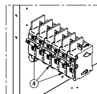
DÉTAIL B
