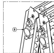
DÉTAIL D
