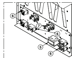
DÉTAIL C
